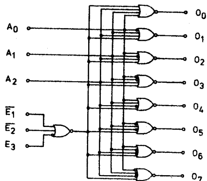
Schemat logiczny
